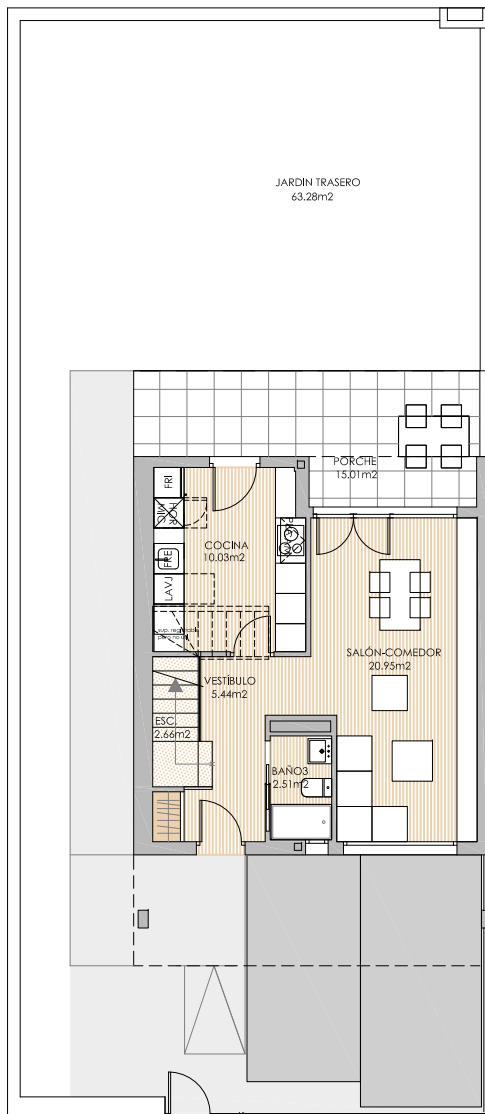
PLANTA BAJA
